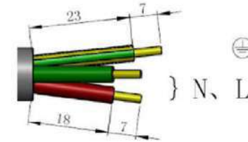
Figura 4.15 Cavi AC tolti
