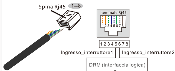
Figura 4.28 Spellare lo strato isolante e collegarlo alla spina RJ45
