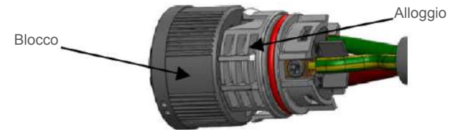
Figura 4.16 Connettere i Cavi al Terminale
